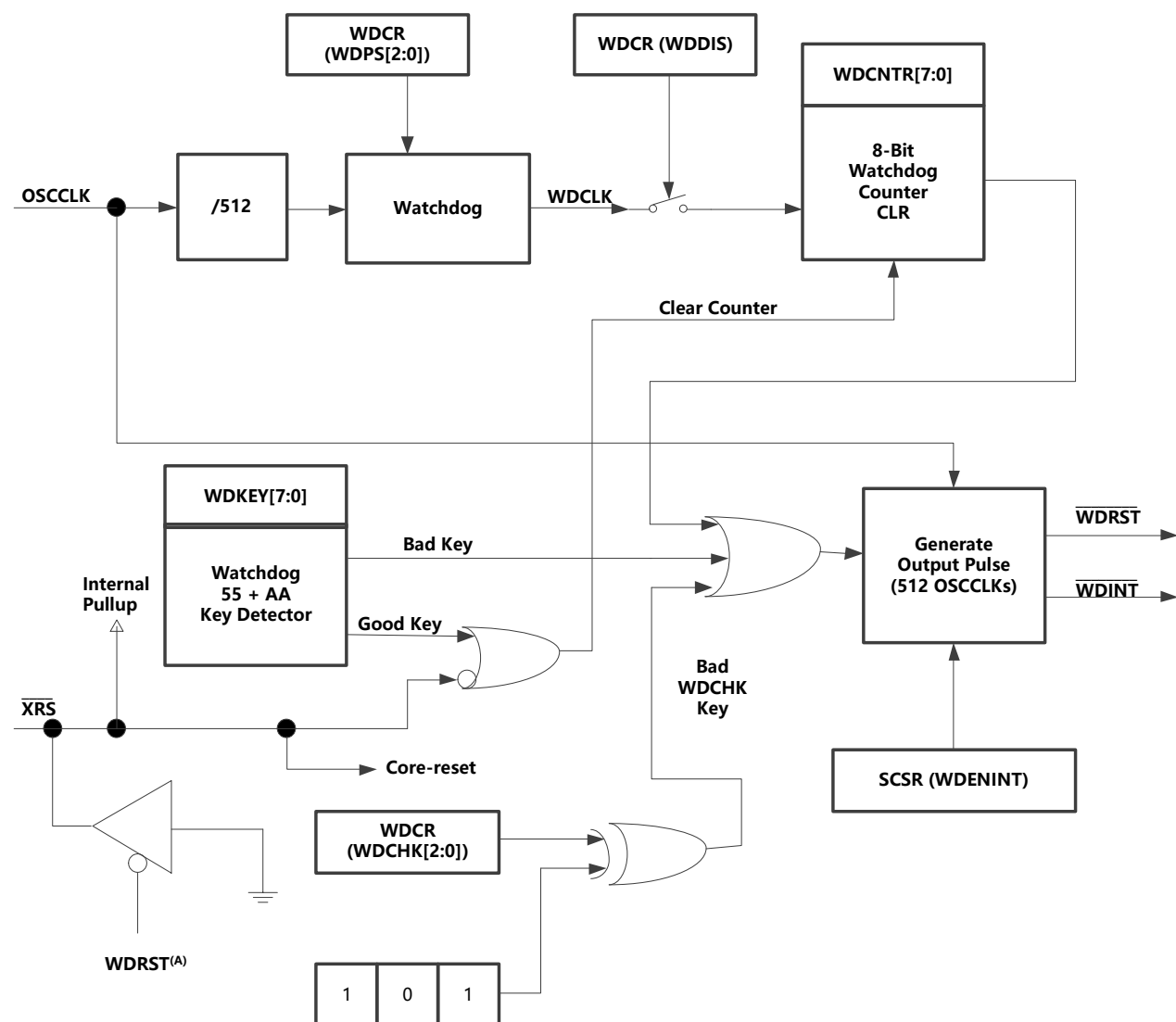
图 2.11 看门狗模块
