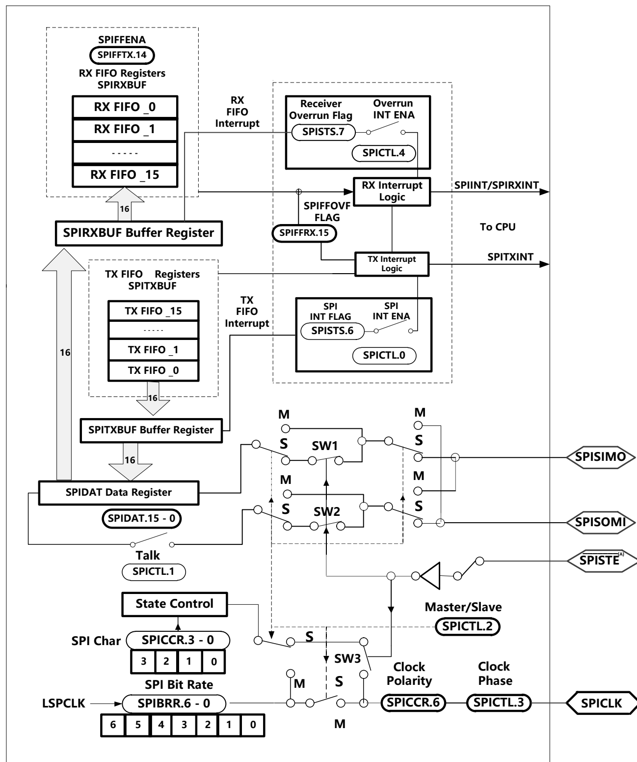
图3-7是一个处于受控模式下的SPI 的方框图。
