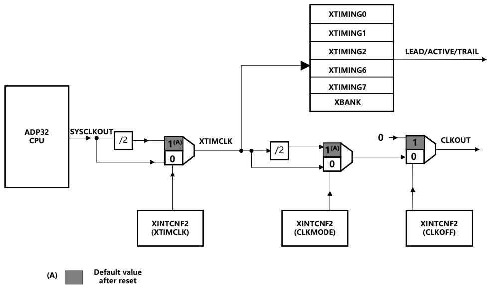
图 5-30. XTIMCLK 和 SYCLKOUT 之间的关系
