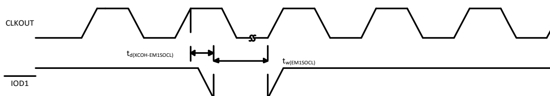
图 5-20. IOD1时序
