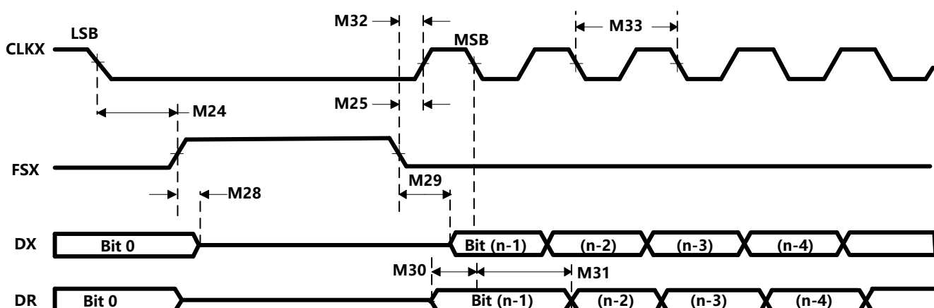
图 5-45. 作为 SPI 主控或者受控时的 McBSP 时序: CLKSTP=10b, CLKXP=0
