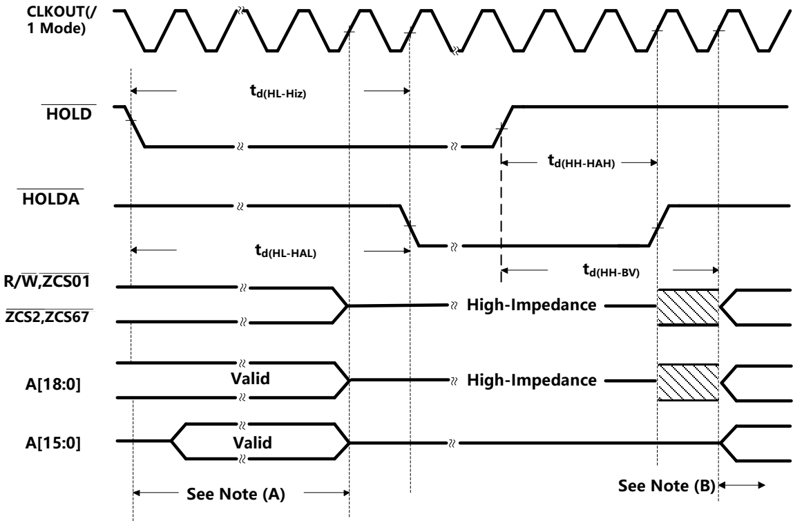
图 5-37. 外部接口保持波形
