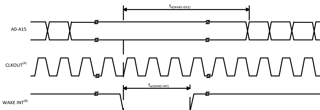
图5-15. IDLE 进入和退出时序
