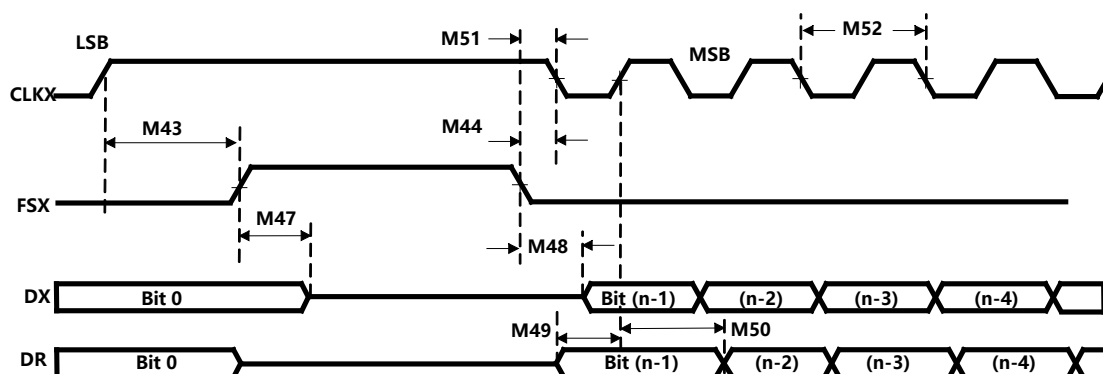
主控或者受控时的McBSP 时序 : CLKSTP= 10b , CLKXP= 1
