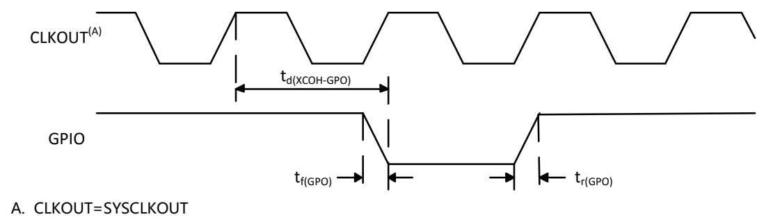
图 5-23. 通用输出时序
