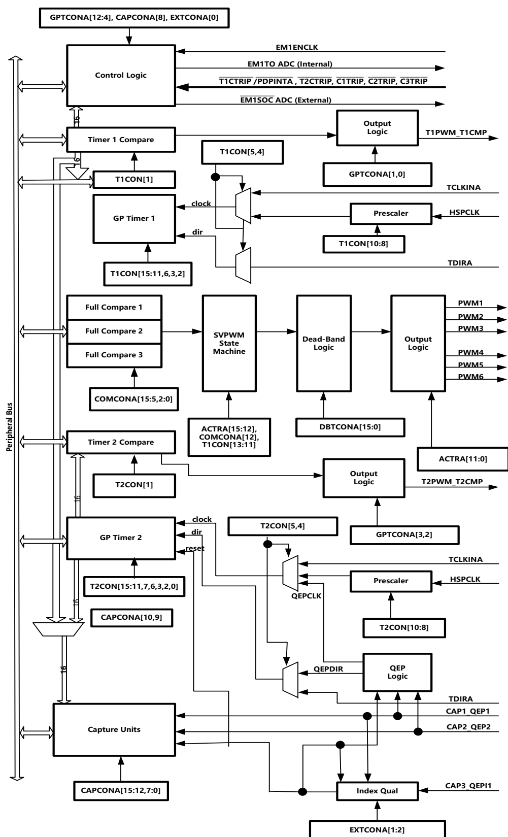
图 3-2. 事件管理器 A 功能方框图
