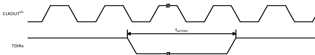
图 5-19.TDIRx 时序
