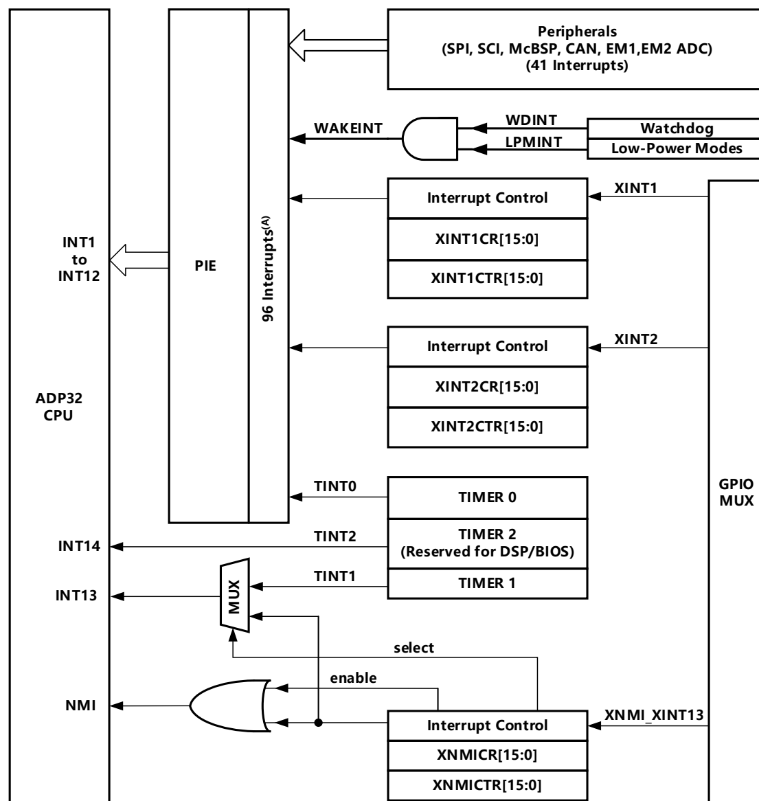
图 2.6-1 中断源
