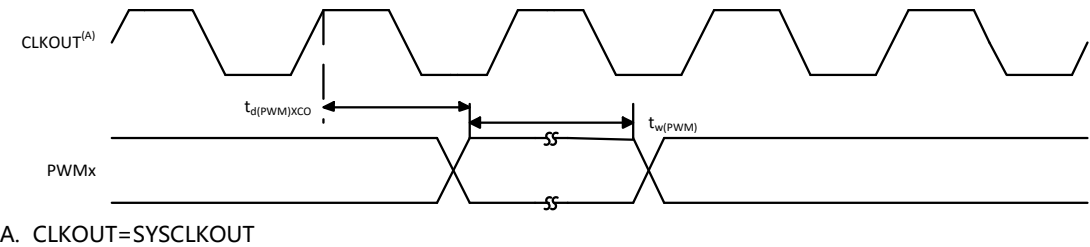
图 5-18.PWM 时序
