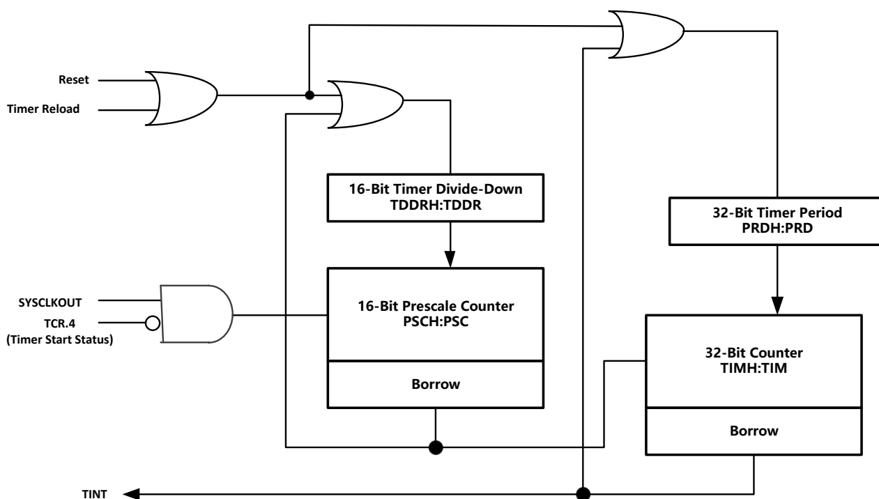
图 3-1. CPU 定时器
