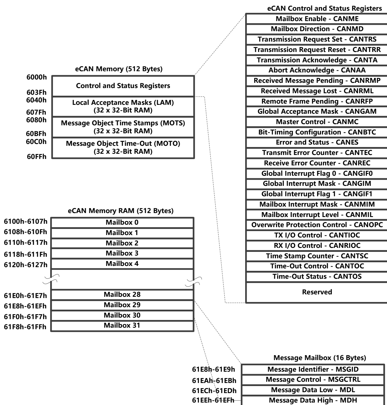
图3.4-2.eCAN内存映射
