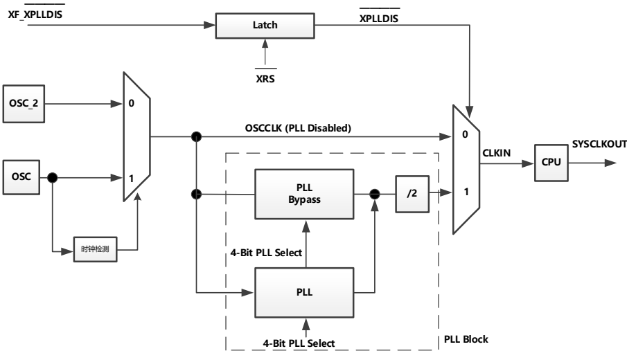
图 2.8-1 OSC 和 PLL 块
