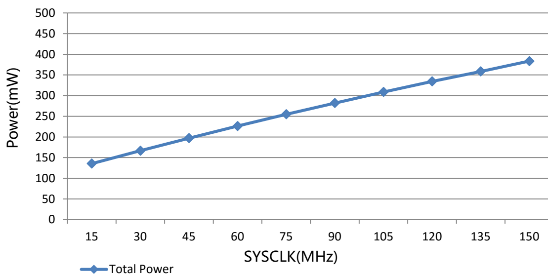
图 5-2. ADP32FXX 在频率范围内的典型流耗
