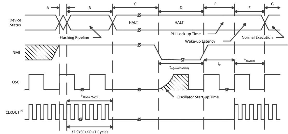
图 5-17. 使用 NMI 的 HALT 唤醒
