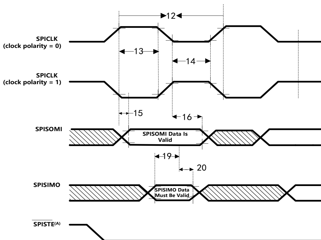
图5-28. SPI 受控模式外部时序 ( 时钟相位= 0 )
